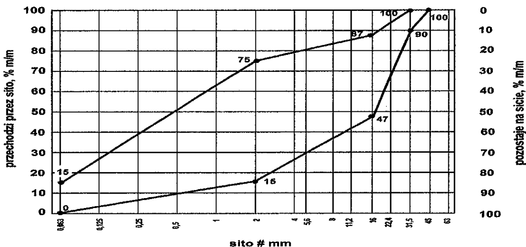
Rys. 3. Krzywe graniczne uziarnienia mieszanki kruszywa niezwiązanego 0/31,5 mm do nawierzchni
