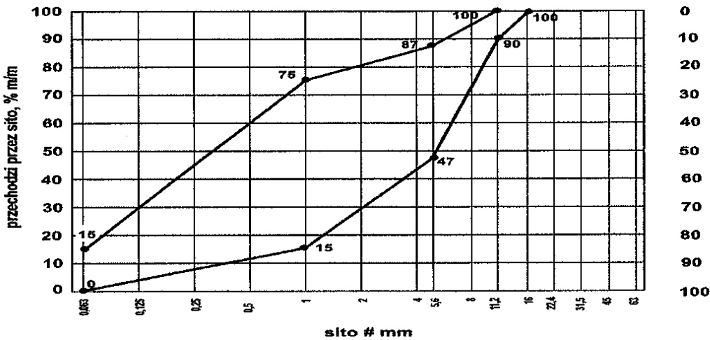
Rys. 1. Krzywe graniczne uziarnienia mieszanki kruszywa niezwiązanego 0/11,2 mm do nawierzchni
