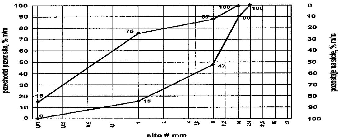
Rys. 2. Krzywe graniczne uziarnienia mieszanki kruszywa niezwiązanego 0/16 mm do nawierzchni
